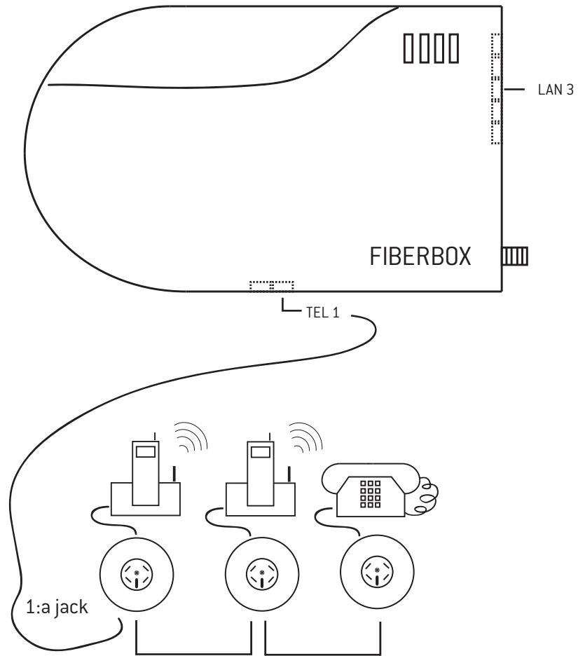
FRÅN FIBERBOX TILL 1:A JACKET
